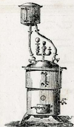
Chaudière à vapeur avec sa bouteille d'alimentation.
