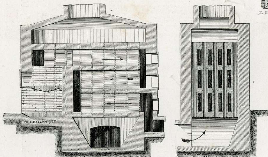
Calorifères en terre réfractaire avec enveloppe en briques.
